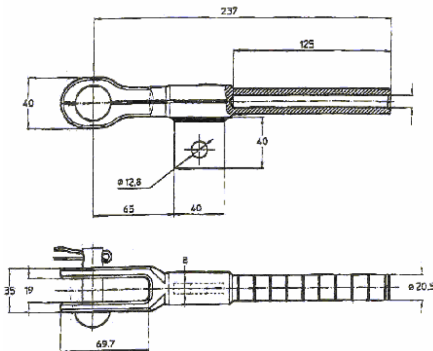
Анкерный зажим A50R+TR, установленный на системе СИП 22 кВ типа DISTRI
