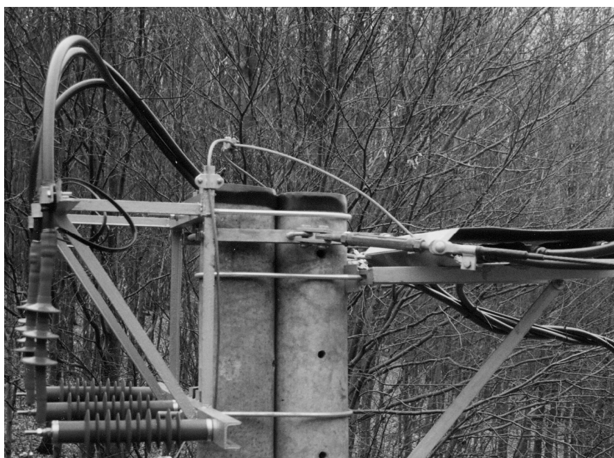
Ответительные муфты на линии СИП до 42 кВ
