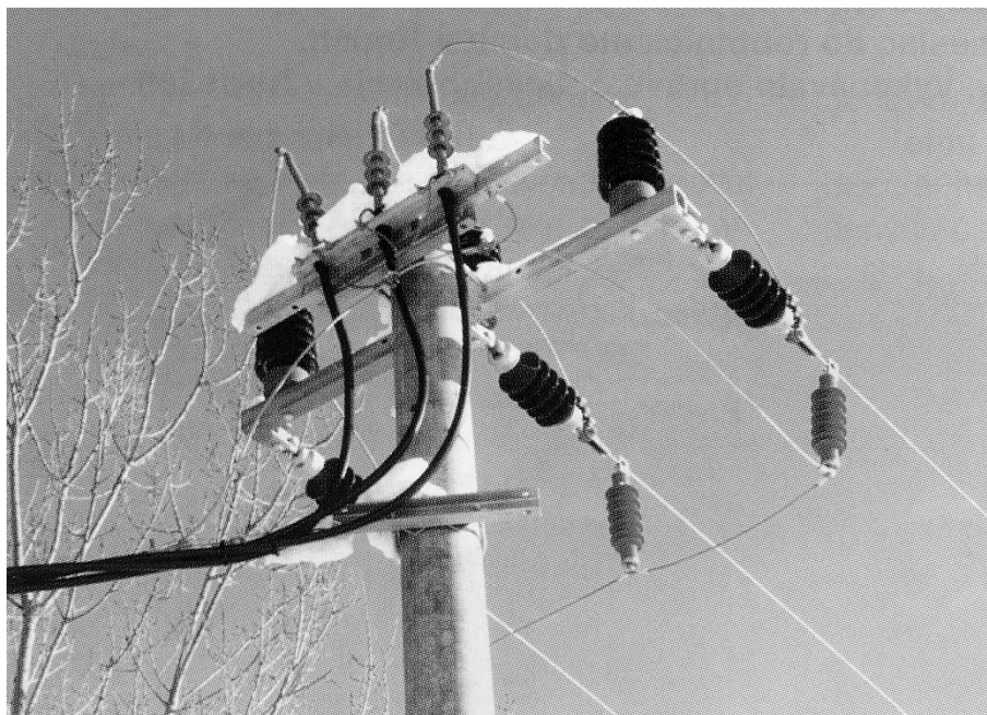
Переход линии СИП среднего напряжения к голым проводам, защищенный металлооксидными ОПН типа HDA-24NA-NLP
