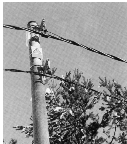
Линии СИП до 42 кВ и до 1 кВ на одной опоре
