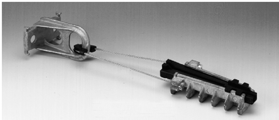
Комплект анкерного зажима ЕА2000, состоящий из кронштейна СА и анкерного зажима РА 2000
